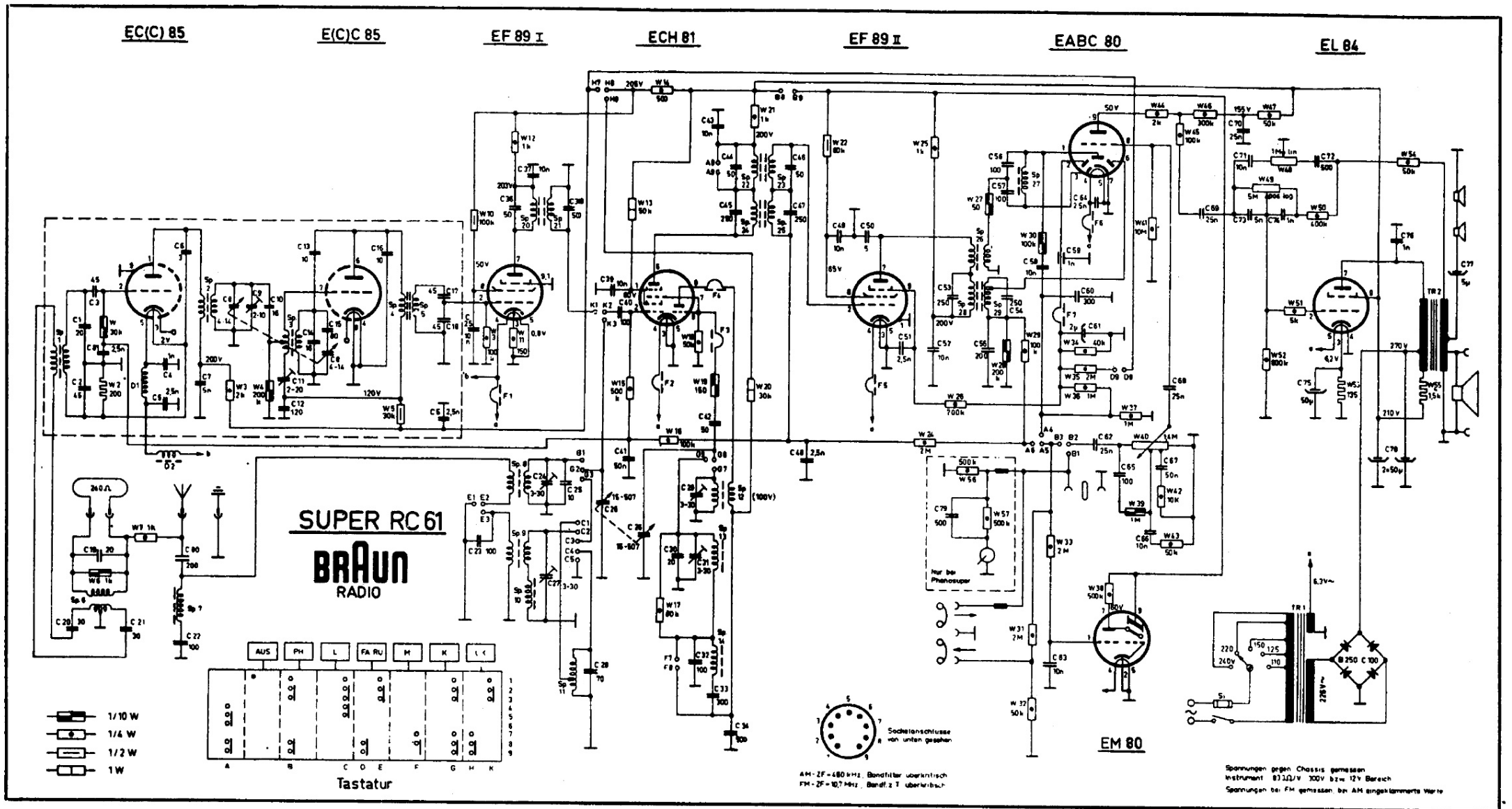
BRAUN (Max Braun Werke, Frankfurt/Main) - Mod. RC61. Apparecchio a modulazione di ampiezza e di frequenza. Gamma onde lunghe, gamma onde medie e gamma onde corte. Gamma onde ultracorte FM. Medie frequenze a 460 kc/s e a 10,7 Mc/s. Potenza d'uscita 3 watt. Consumo 50 watt.
